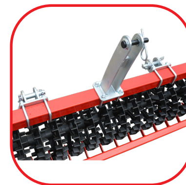
3-PUNKTOWY ZACZEP DREIPUNKTAUFHÄNGUNG THREE-POINT HITCH
